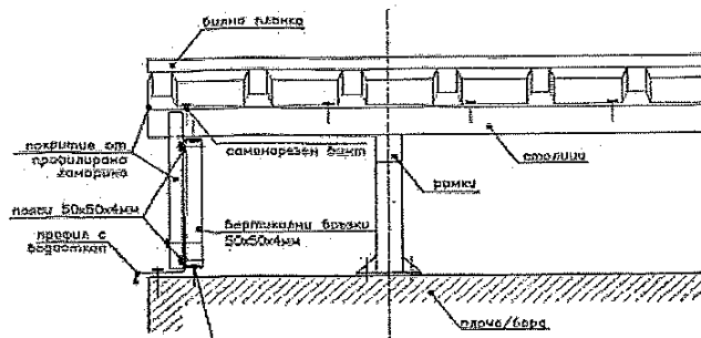
стенова ферма с професи 50x50x4mm и покритие от профилна ламарина за затваряне на отвор
