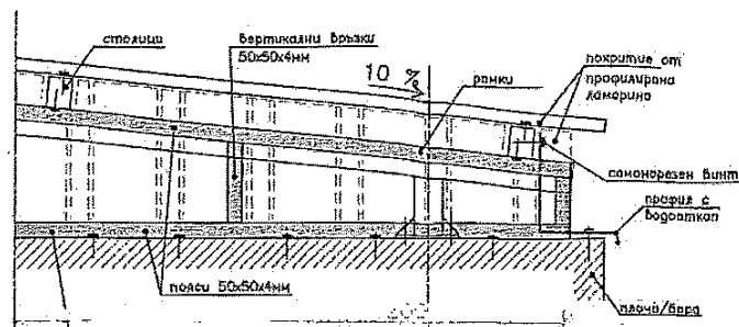
стенова ферма с професи 50x50x4mm и покритие от профилна ламарина за затваряне на отвор
