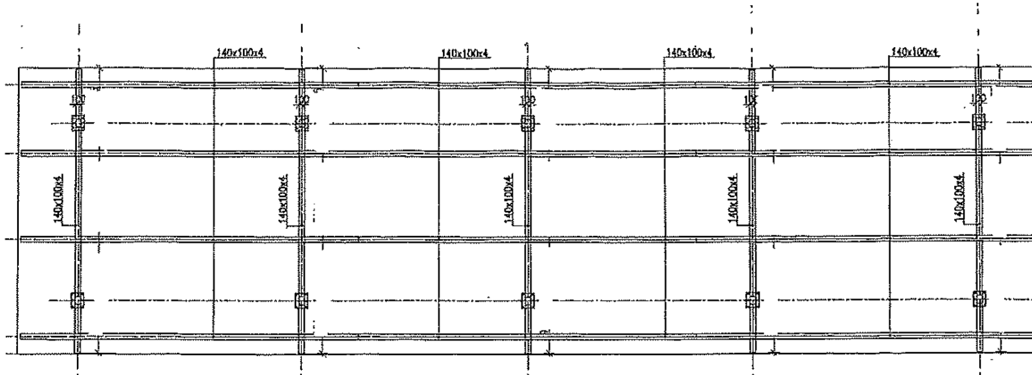
Ферми при крайни рамки за затваряне на отвори при едноскатен покрив
