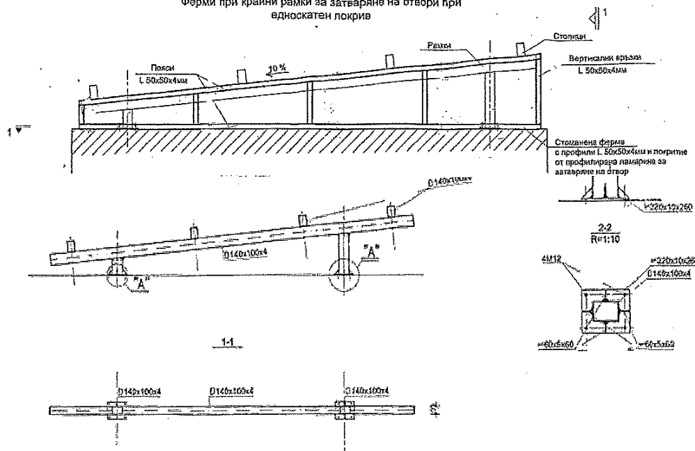
Ферми при крайни рамки за затваряне на отвори при едноскатен покрив
